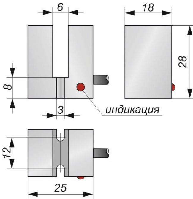
Габаритный чертеж
