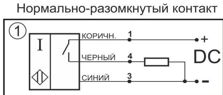
Схема подключения
