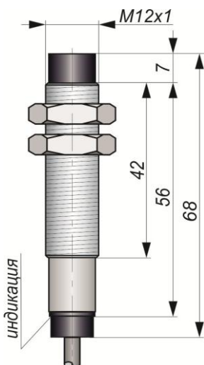
Габаритный чертеж
