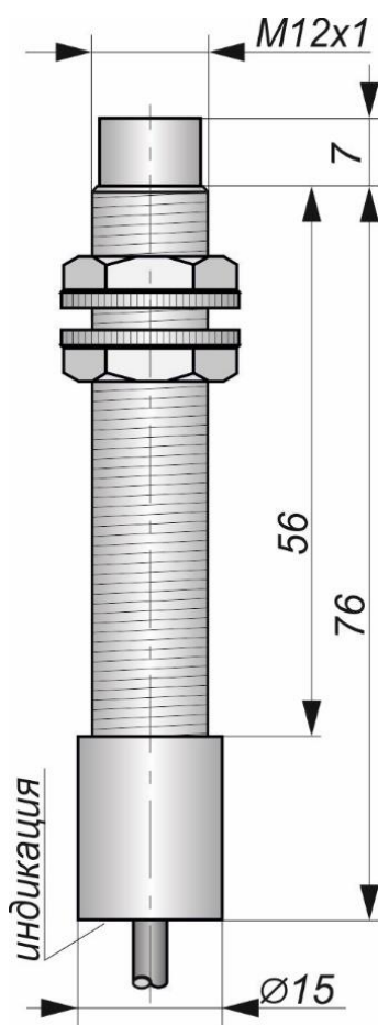
Габаритный чертеж
